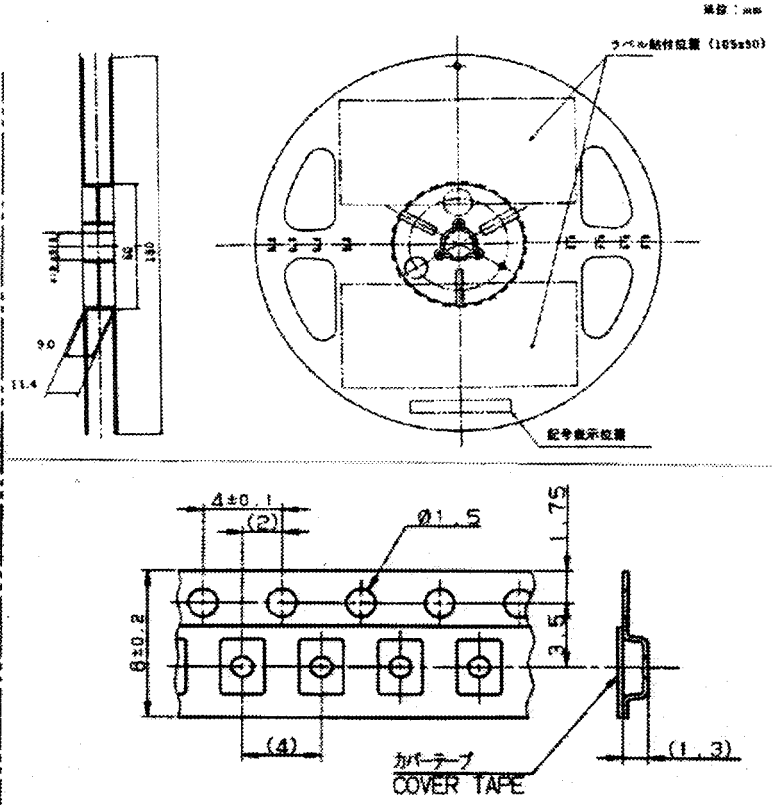
EIAJ規格品 (参考寸法) リール寸法 FIG.2 REEL DIMENSION
