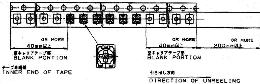
FIG.3 EIAJ規格準拠
