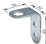
取付L金具 L-52 ¥730
