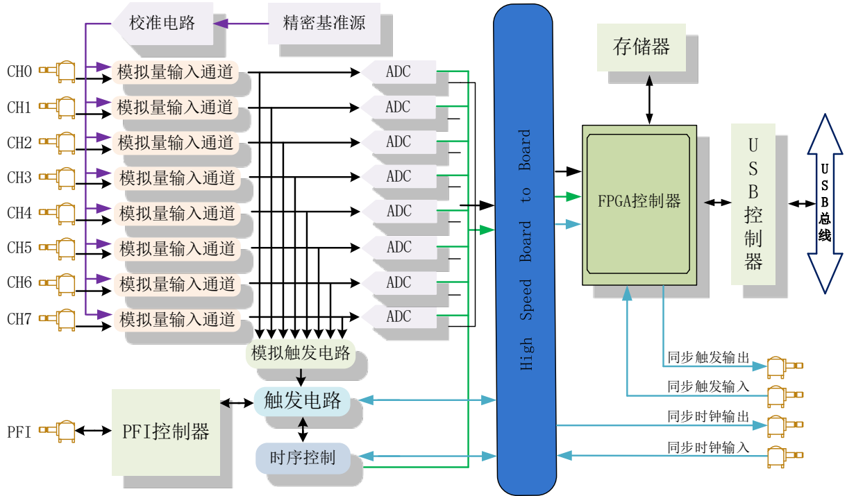
图 3-1-1 USB858X 系统框图
