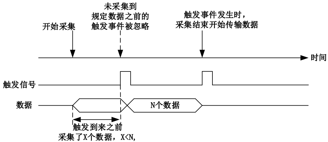
图 4-9-2-6 硬件延时触发
