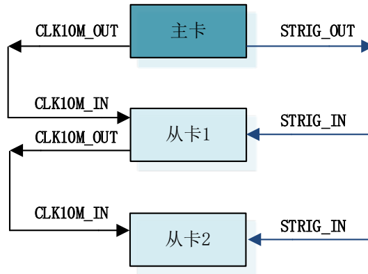
图4-10-1 主从卡级联
