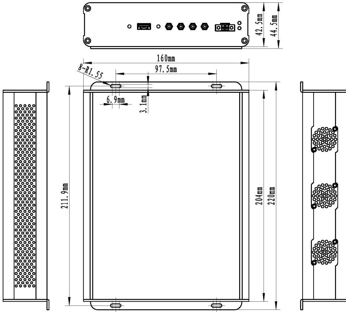
图 3-4-1 USB858X 产品外壳尺寸图
