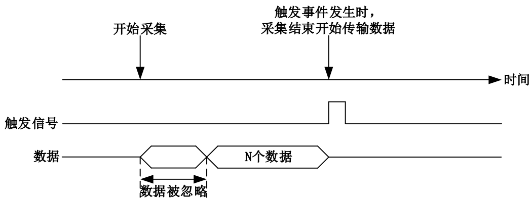
图 4-9-2-4 预触发
