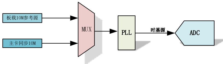
图 4-7-1 时基源框图
