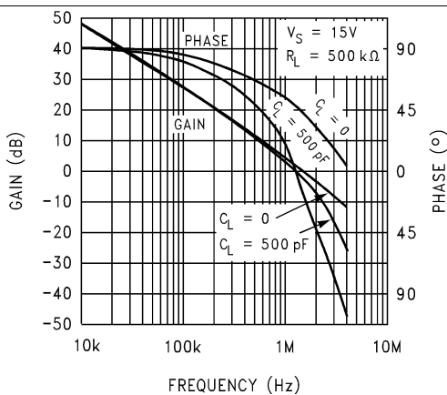
Figure 30. 增益和相位与容性负载间的关系
