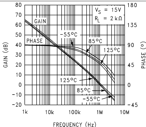
Figure 28. 开环频率响应与温度间的关系
