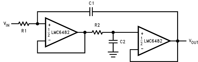
Figure 77. 轨至轨单电源低通滤波器
