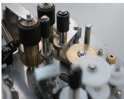
工业级机芯
