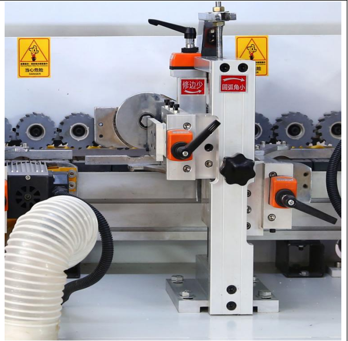
刮边装置
