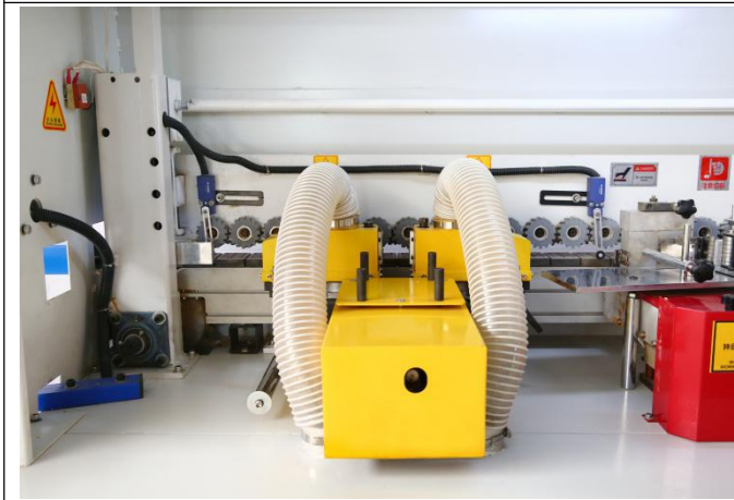
预铣装置
