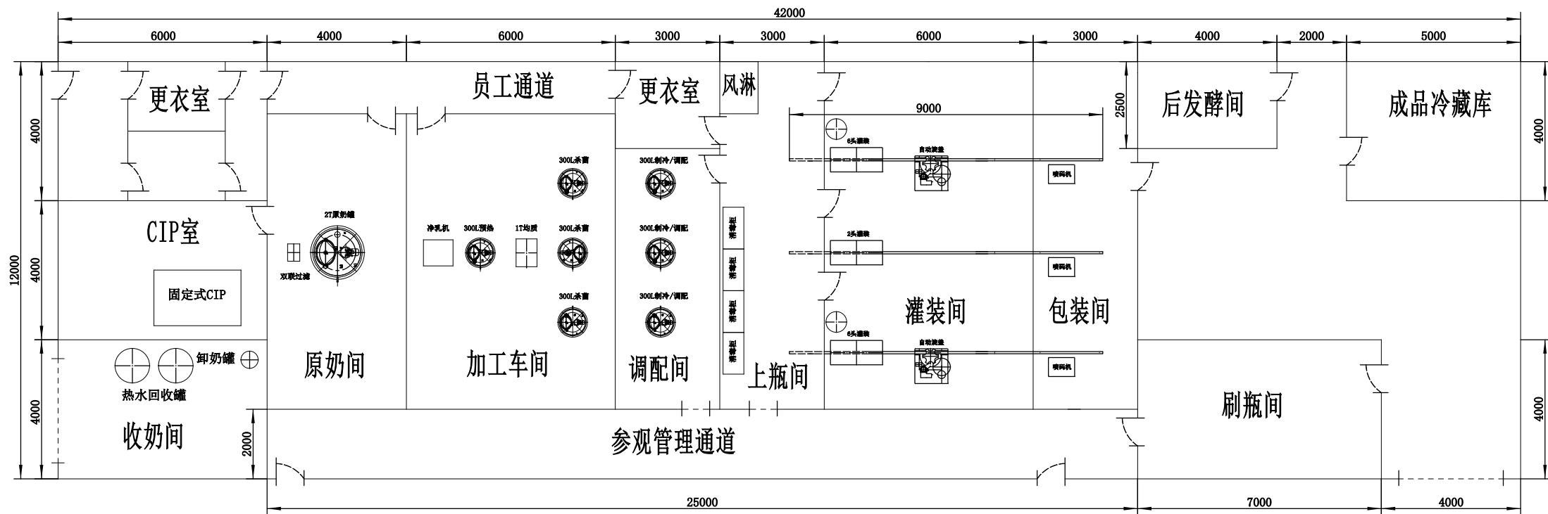
山东美川机械 河南健羊牧业一期羊奶深加工车间布局图
