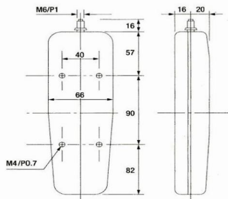
外型尺寸 Outline UNIT/mm
