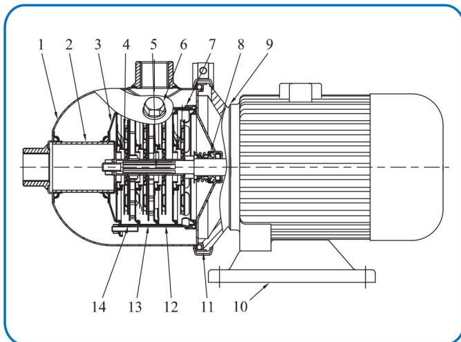
截面图 RV, RVK 2,4
