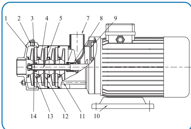
截面图 RVF, RVF (T)
