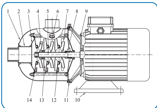
截面图 RV, RVK 8,12,16,20
