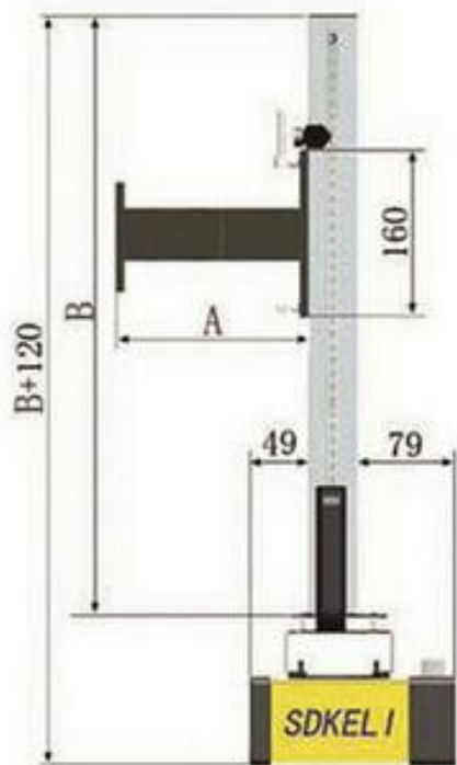
支架装配图 Assembly drawing
