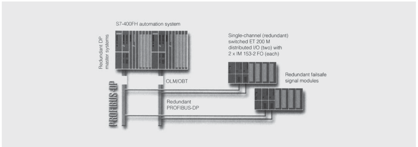
图：冗余切换式 I/O 的配置
