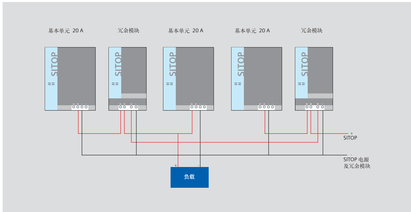
3 台及 3 台以上 20 A 及以内电源并联接线示意图
