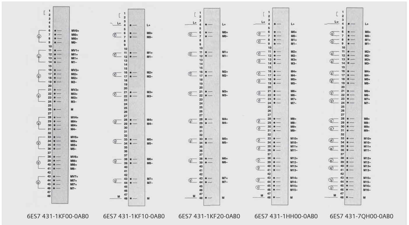
图：用于电压测量的模拟量输入模板的端子接线图
