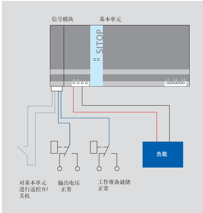
信号模块安装接线示意图
