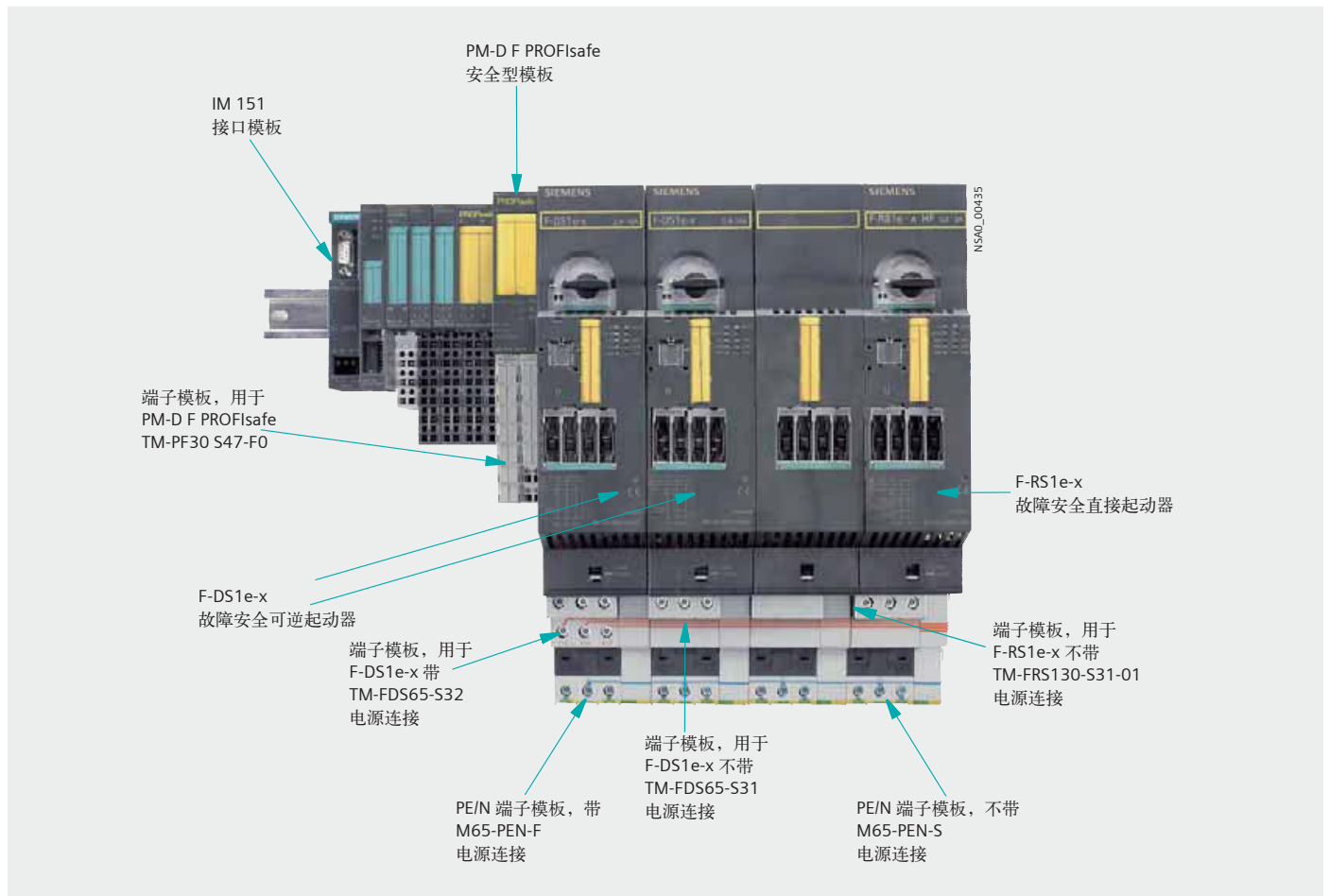
ET 200S 安全型电机起动机解决方案 PROFIsafe 组件的配合使用
