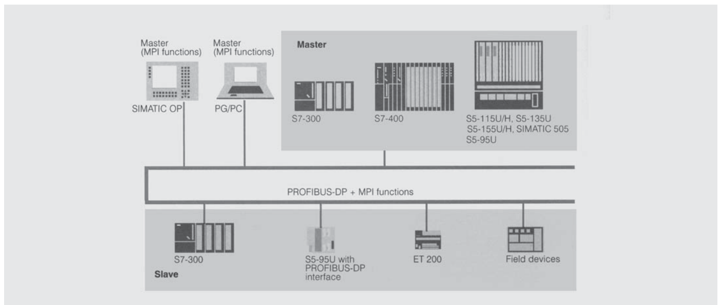
图：应用 PROFIBUS-DP 总线系统的联网
