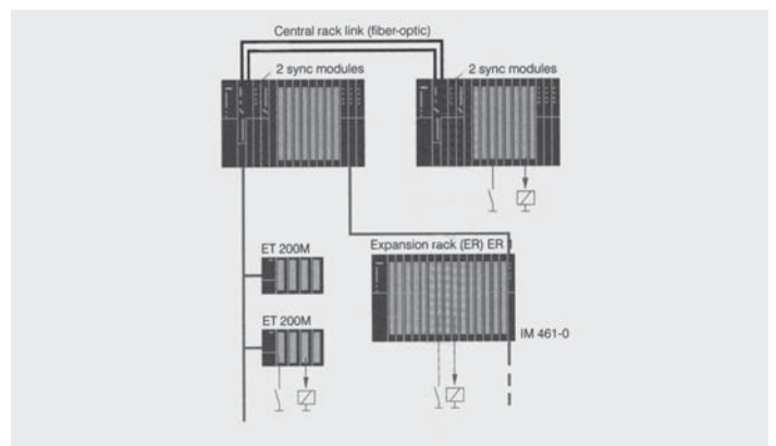
图：单边配置（常规的可用性）
