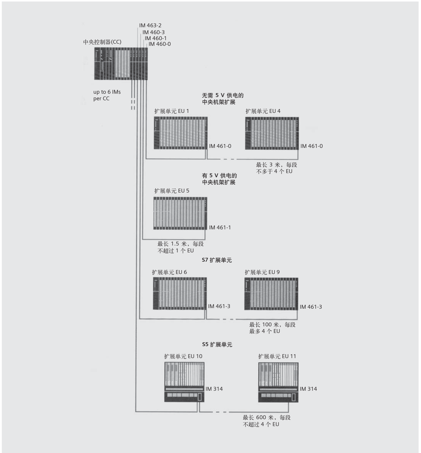
图: S7-400 可能的扩展型式
