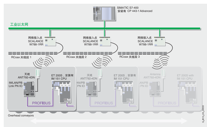
图: 通过快速漫游, 实现 RCoax 电缆网段之间的快速数据传输
