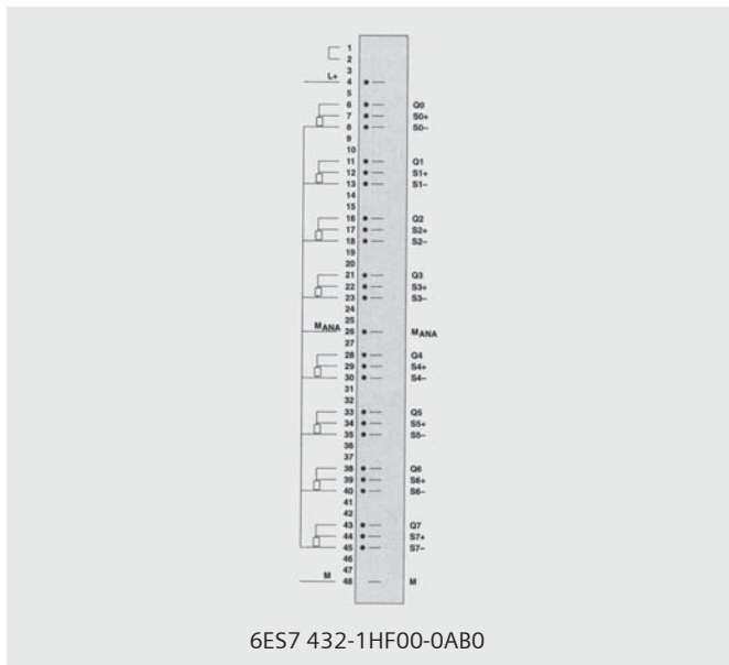
图：模拟量输出模板的端子接线图
