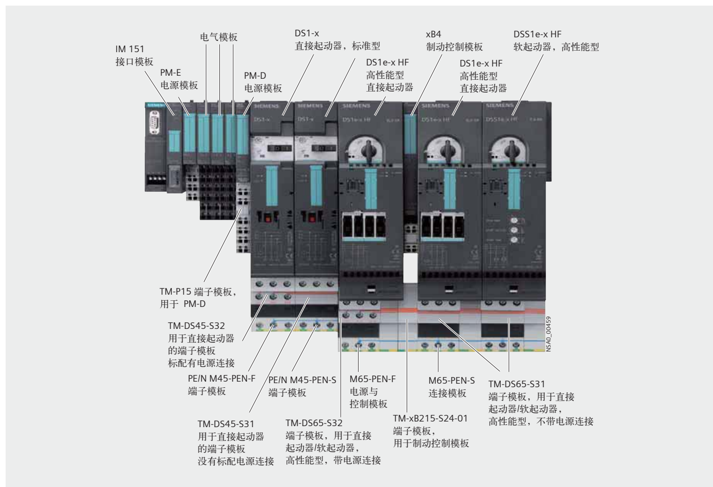
ET 200S 电机起动机组件的配合使用
