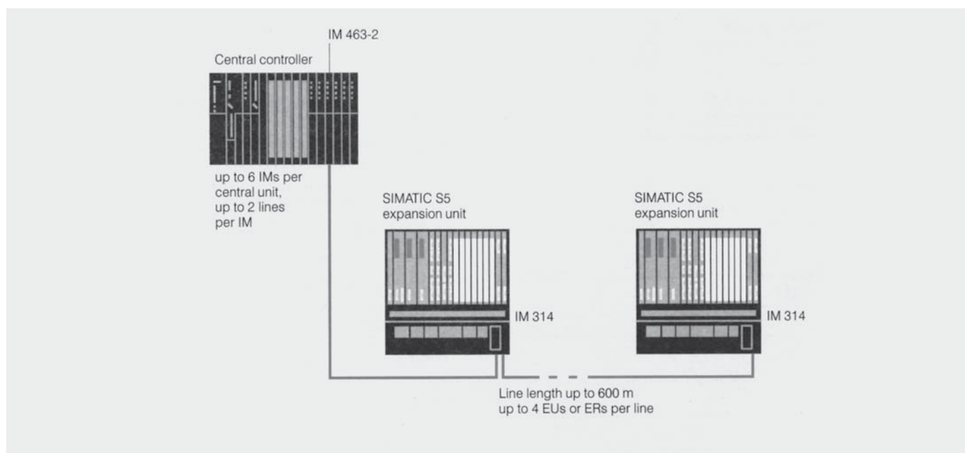
图：用 SIMATIC S5 扩展单元的扩展
