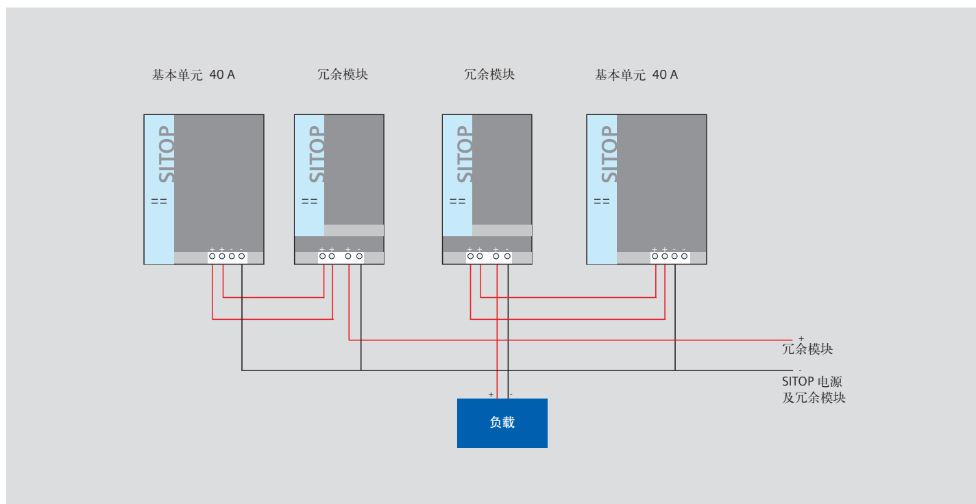
20 A 以上电源并联接线示意图
