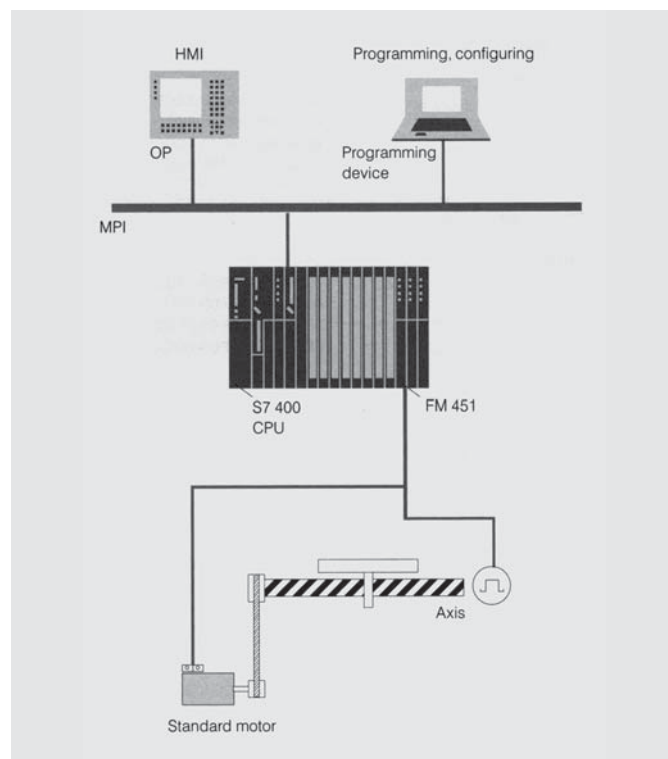
图：使用 FM451 的定位控制
