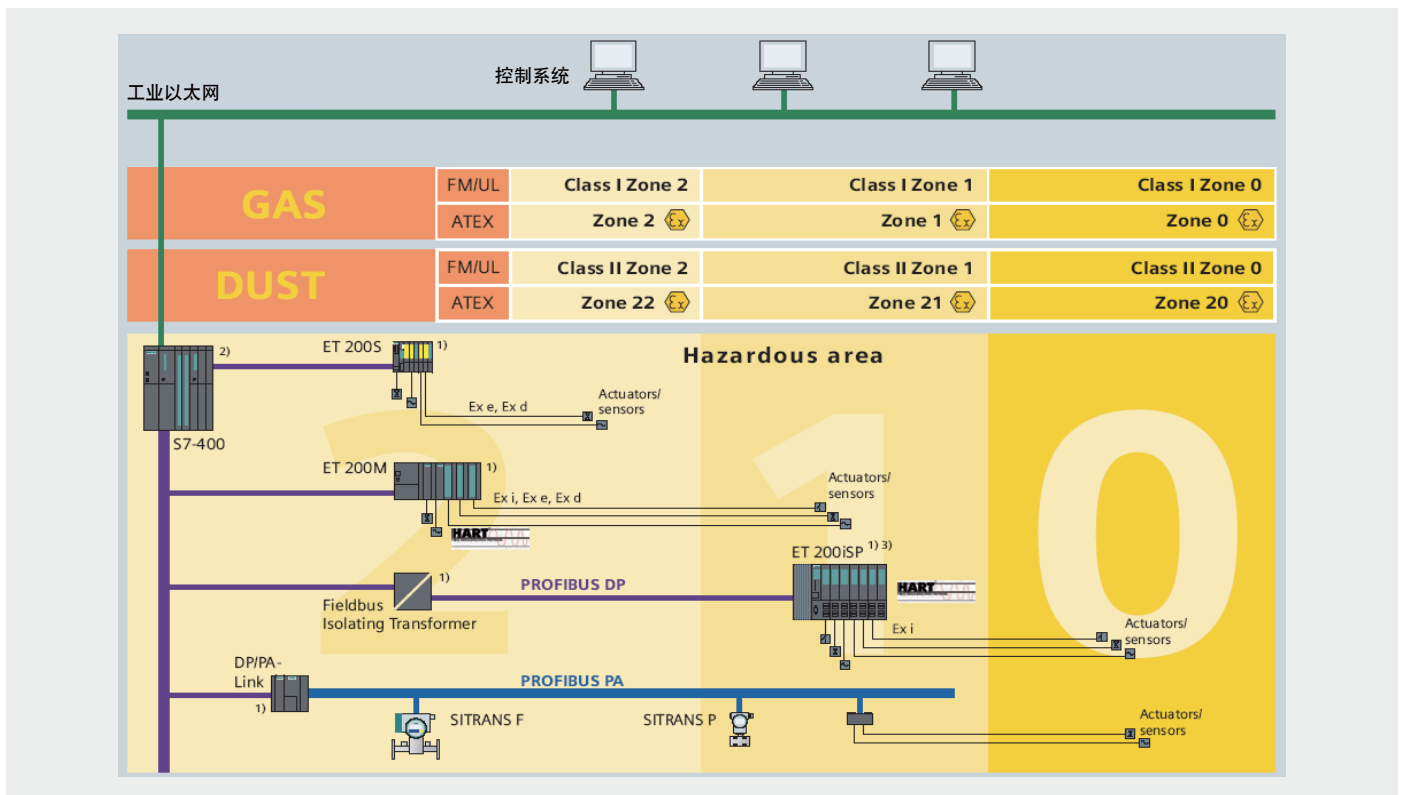
ET 200iSP 在危险气体和粉尘环境下的应用
