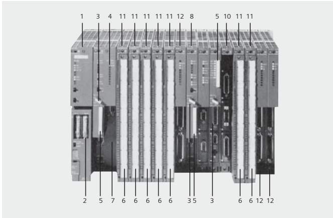
图：使用 CR2 机架的 SIMATIC S7-400 可编程序控制器
