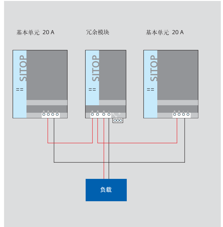
2台 20 A 及以上电源并联接线示意图
