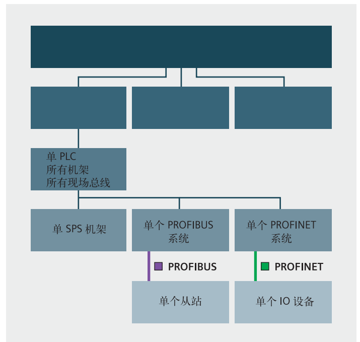
图：SIMATIC 维护站的层级显示
