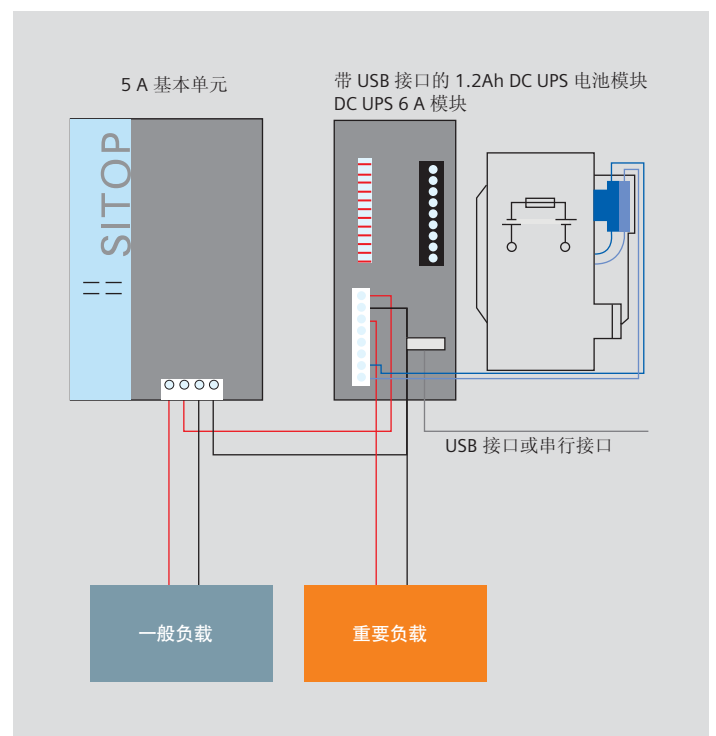
UPS 模块安装接线示意图
