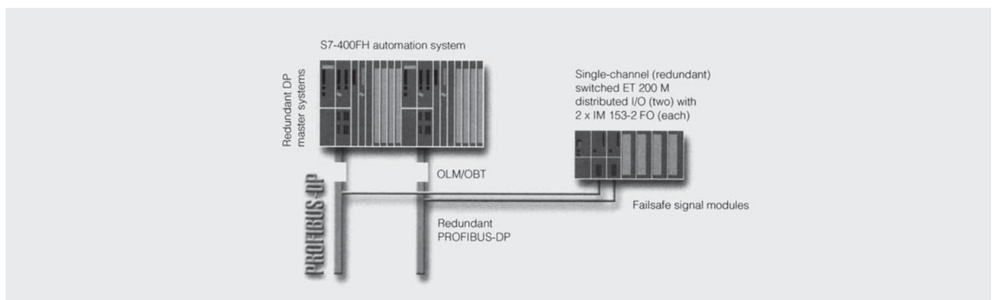
图：单通道、切换式 I/O 的配置
