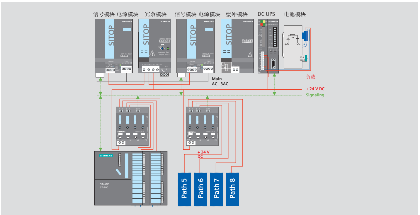
SITOP 电源系统全套解决方案
