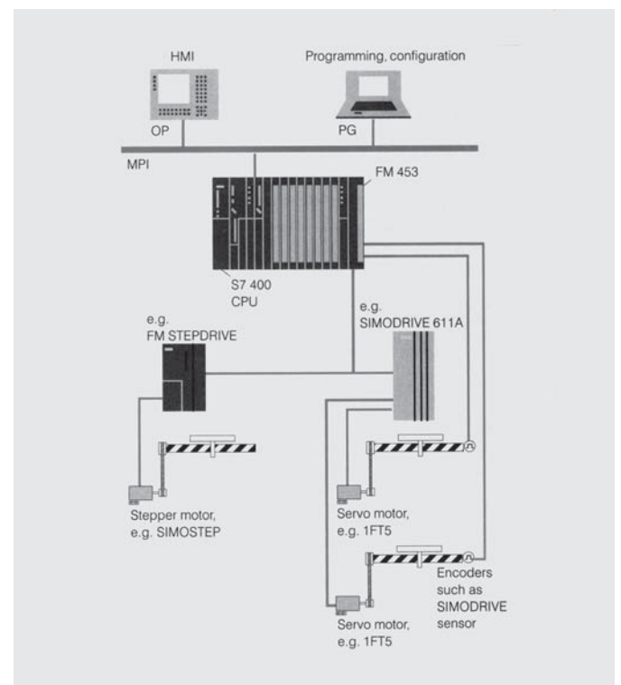
图：用 FM 453 进行定位控制的典型配置
