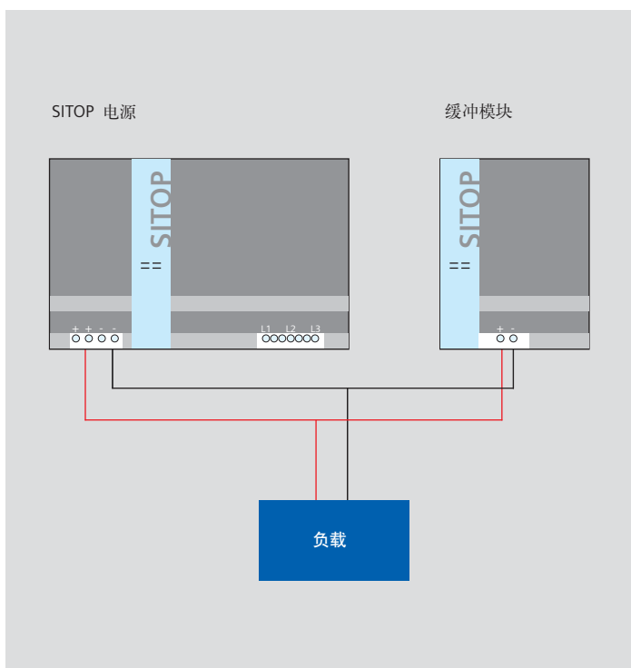
缓冲模块安装接线示意图
