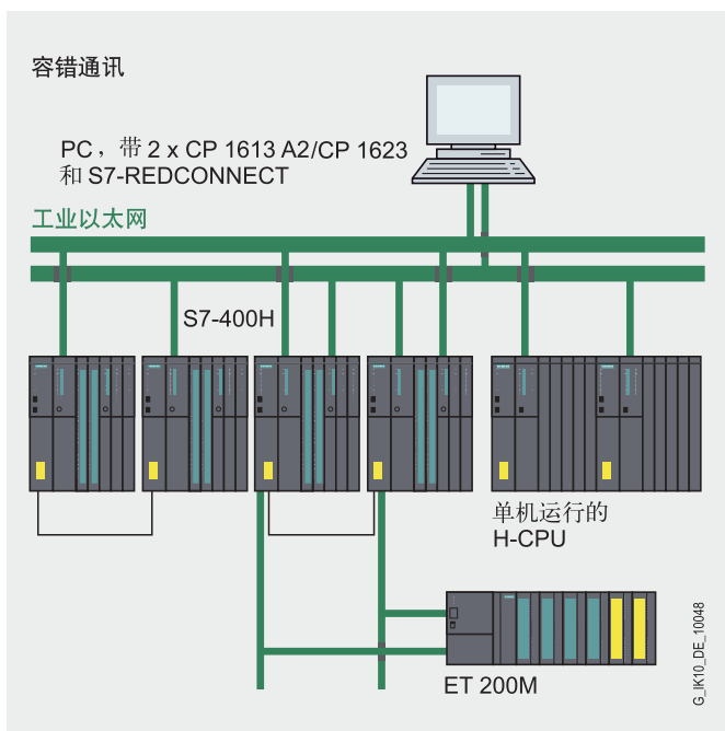
S7-REDCONNECT 系统配置
