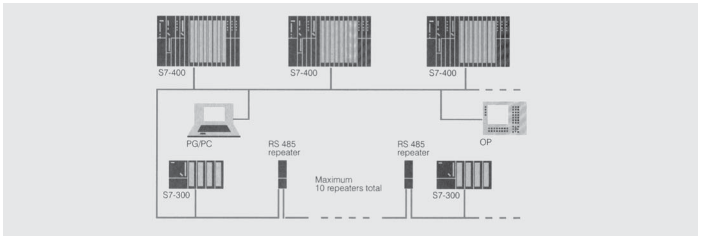
图：典型的带 MPI 接口的通讯配置
