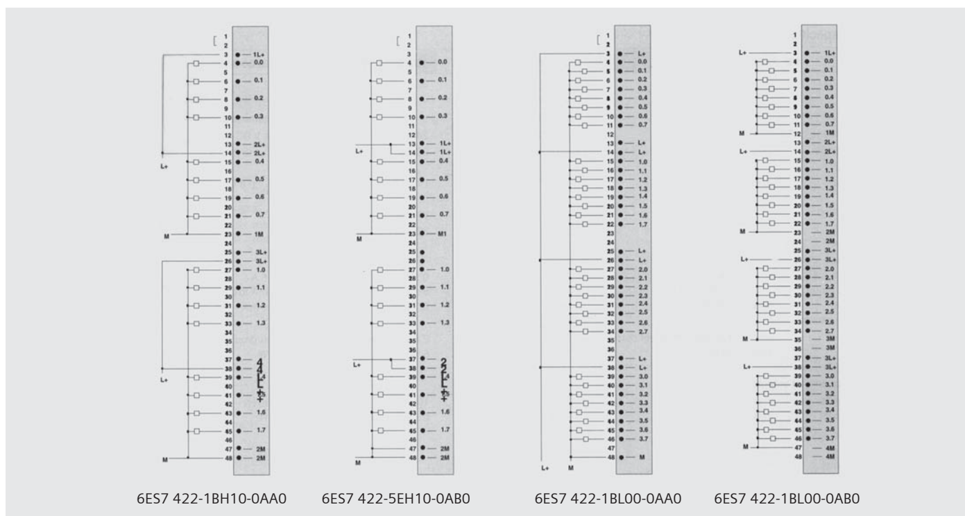
图：数字量输出模板的端子接线图
