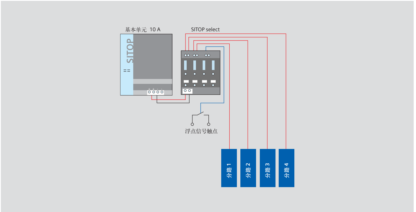
诊断模块安装接线示意图
