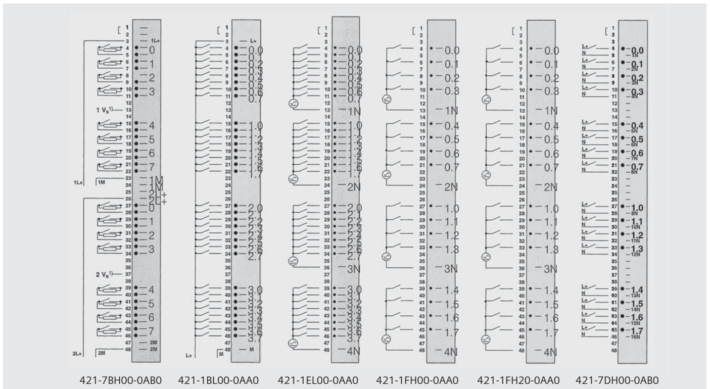
图：数字量输入模板的端子连接图
