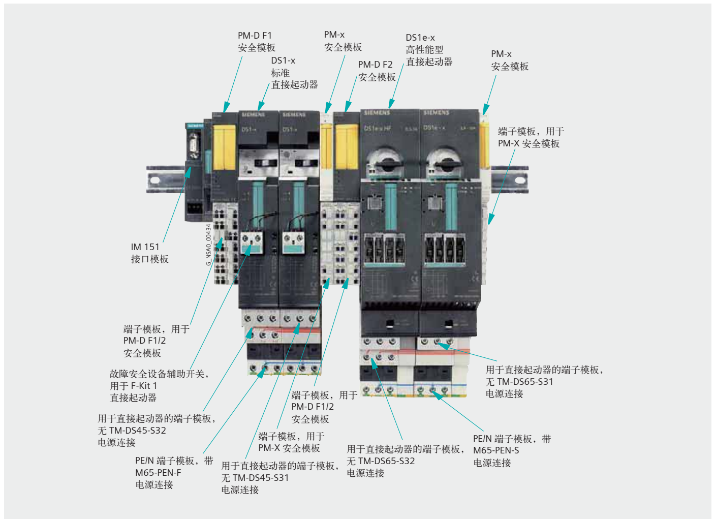
ET 200S 安全型电机起动器解决方案本地组件的配合使用
