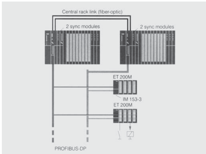
图：切换式配置
