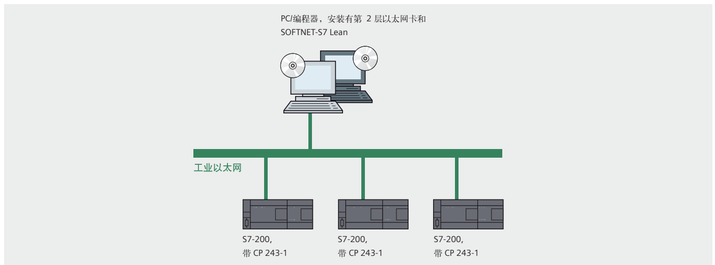
图：采用用于工业以太网的 SOFTNET-S7 Lean 和 S7-200 的系统配置
