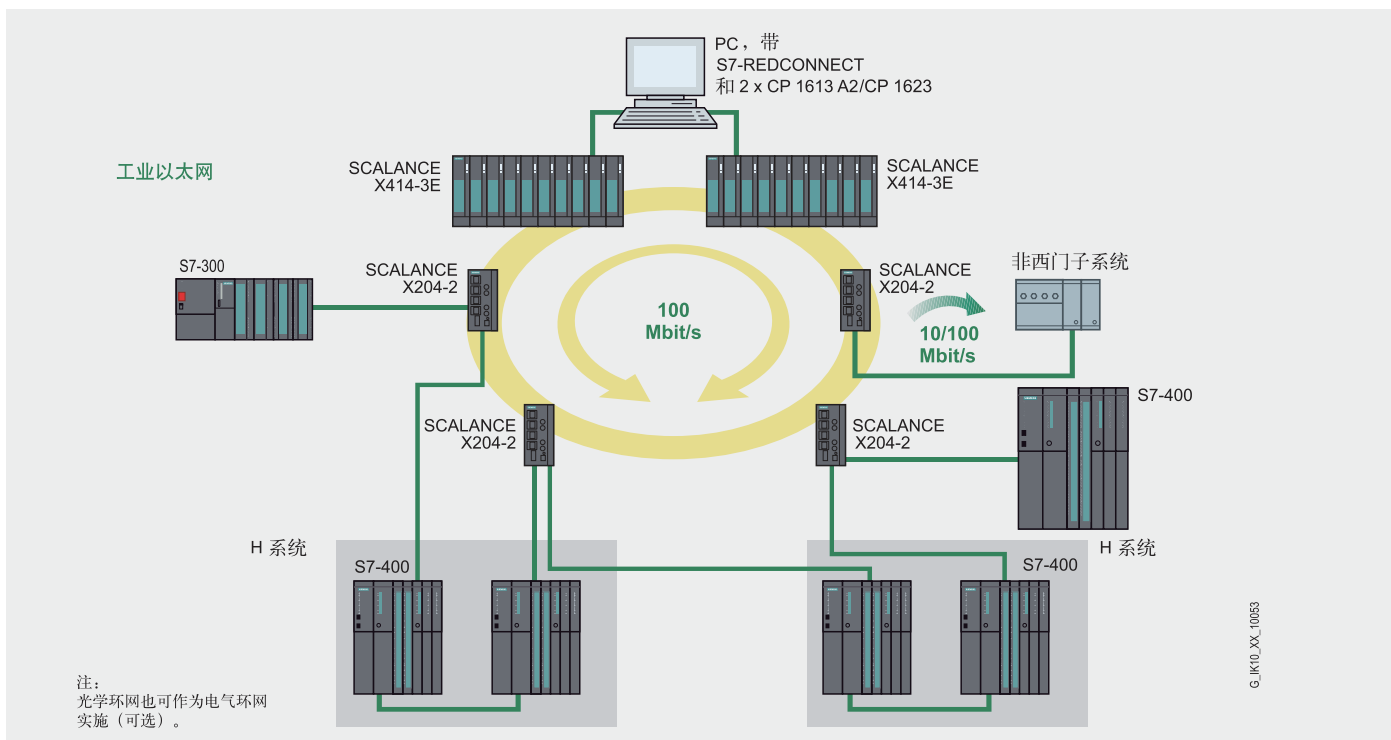
图：通过冗余的环网结构，因而网络具有极高的可用性。
