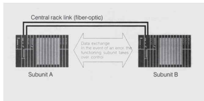
图：S7-400H 的容错通讯
