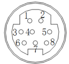
Mini Din 8 芯插座（孔）
