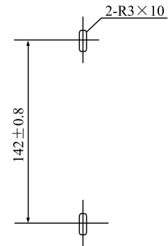
板前接线开孔
