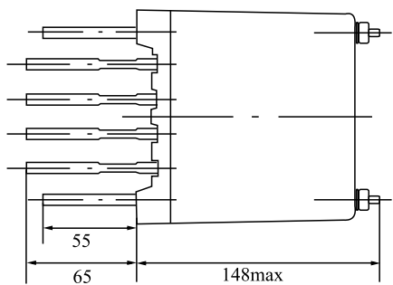
板前接线
