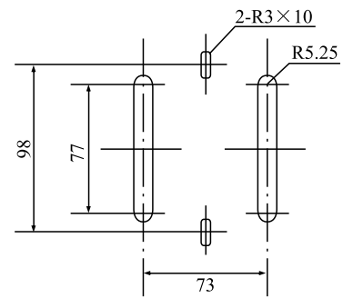
板后接线开孔
