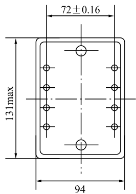
板后接线
