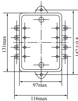
板前接线
